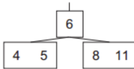
Figura 11: Árbol B
