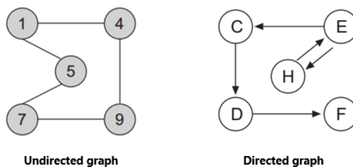
Figura 31: Tipos de grafos
