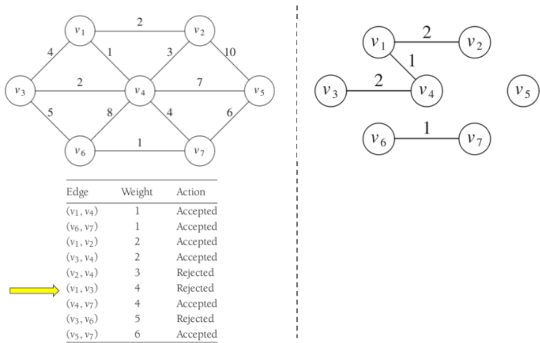
Figura 51: Kruskal
