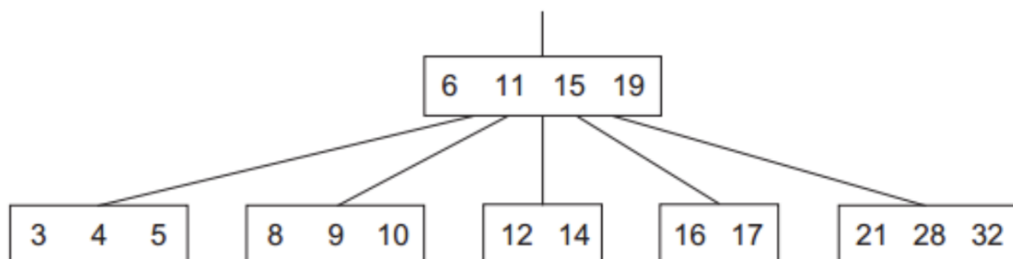
Figura 13: Árbol B
