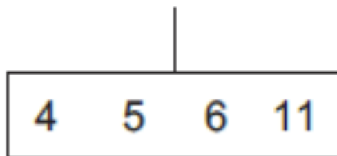
Figura 10: Árbol B
