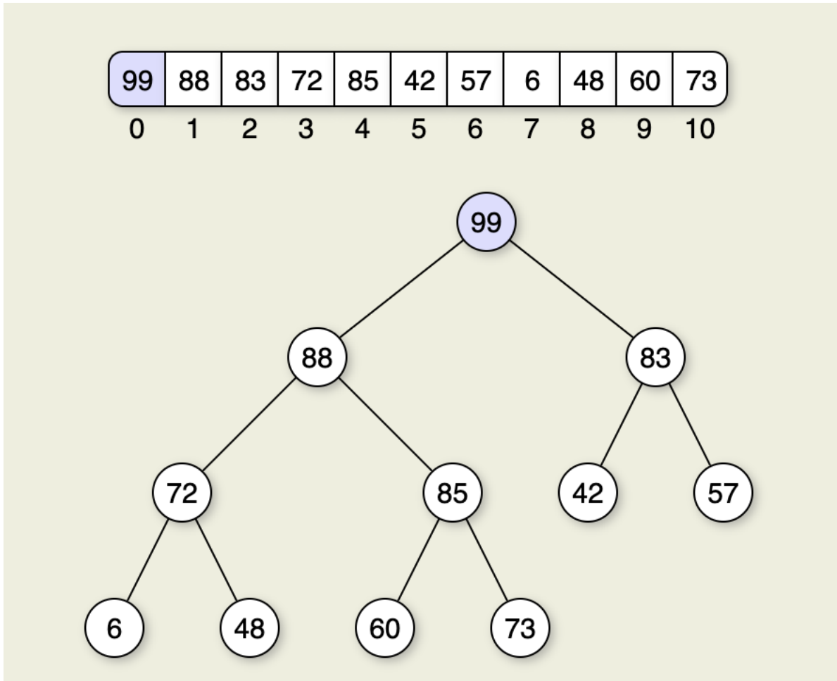
Figura 8: Árbol Heap
