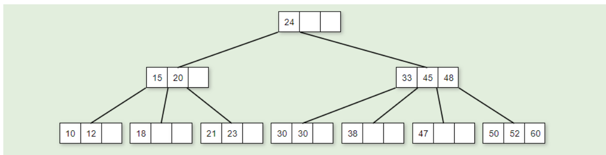
Figura 9: Árbol B
