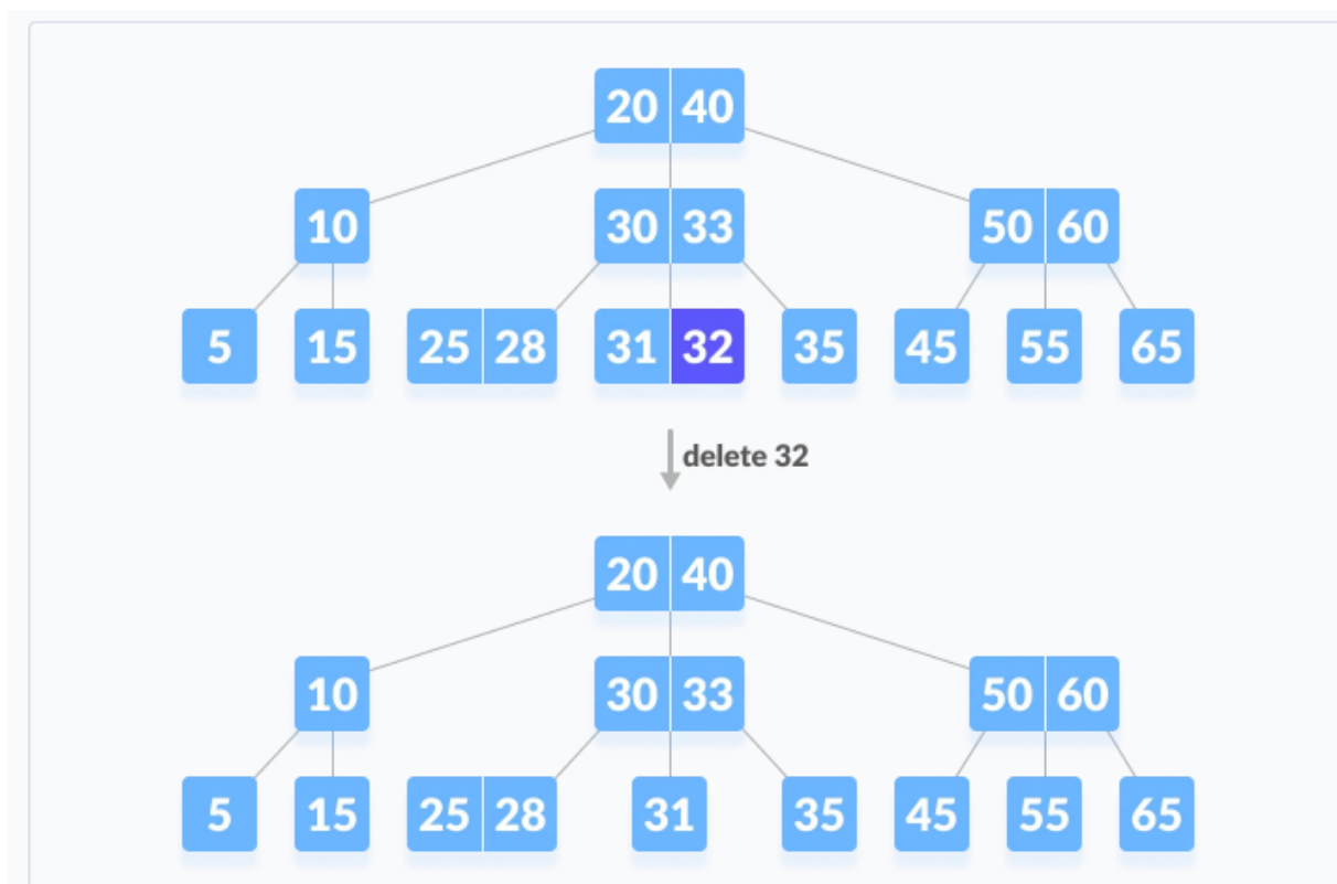
Figura 14: Árbol B
