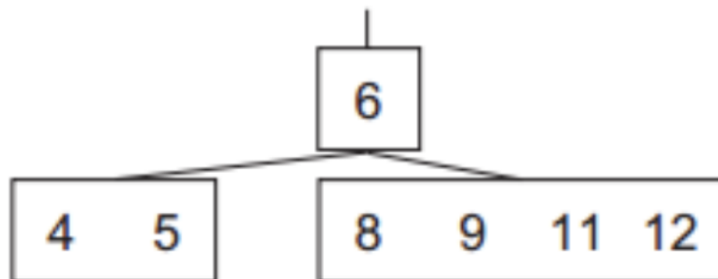
Figura 12: Árbol B
