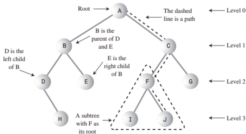
Figura 6: Árbol binario
