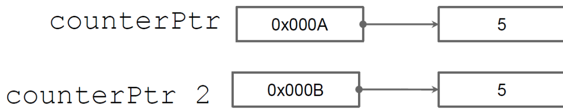
Figura 16: Deep copy
