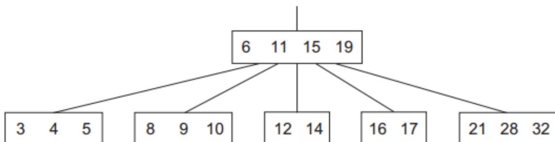
Figura 13: Árbol B
