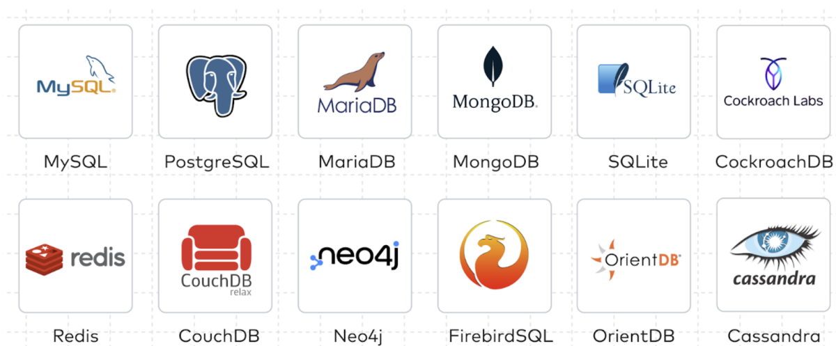
Figura 28: DBMS populares
