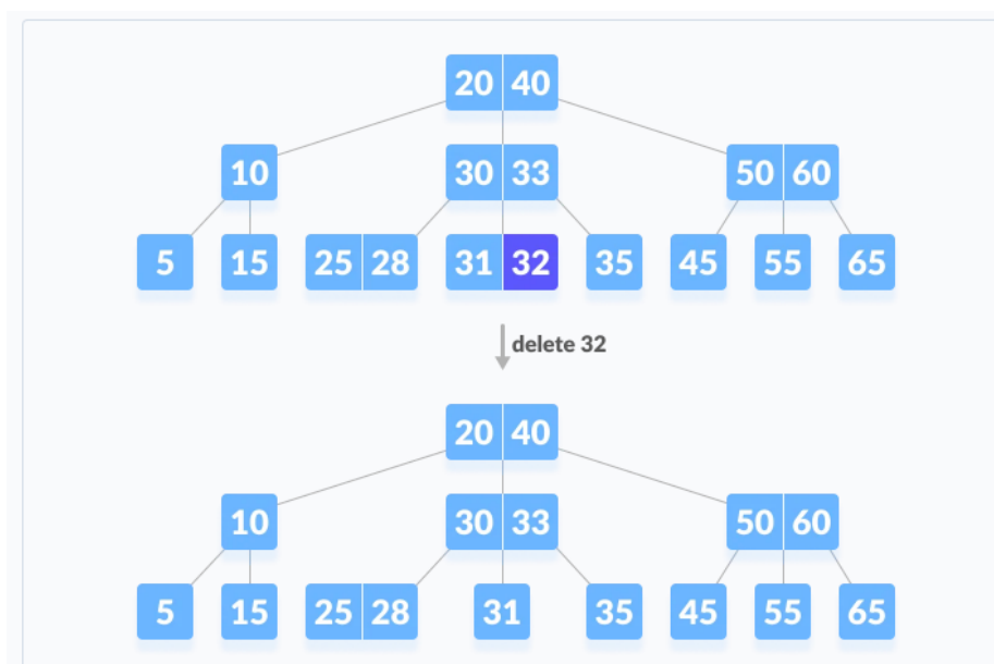
Figure 3.9: Árbol B
