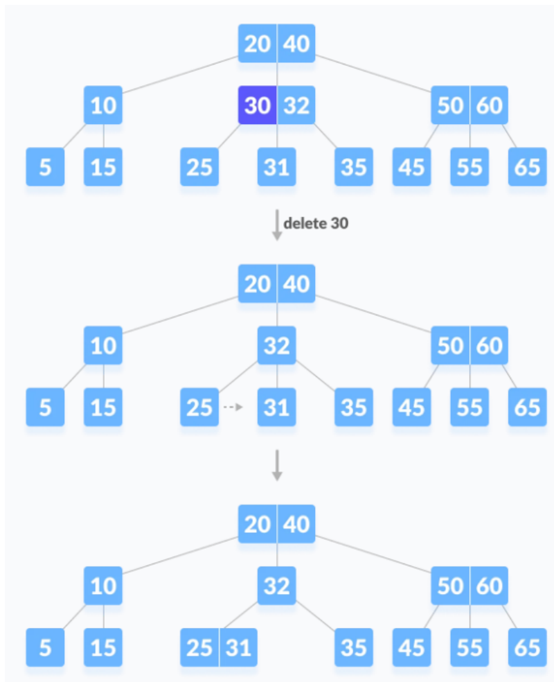
Figure 3.13: Árbol B
