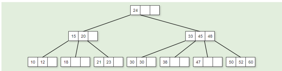
Figure 3.4: Árbol B
