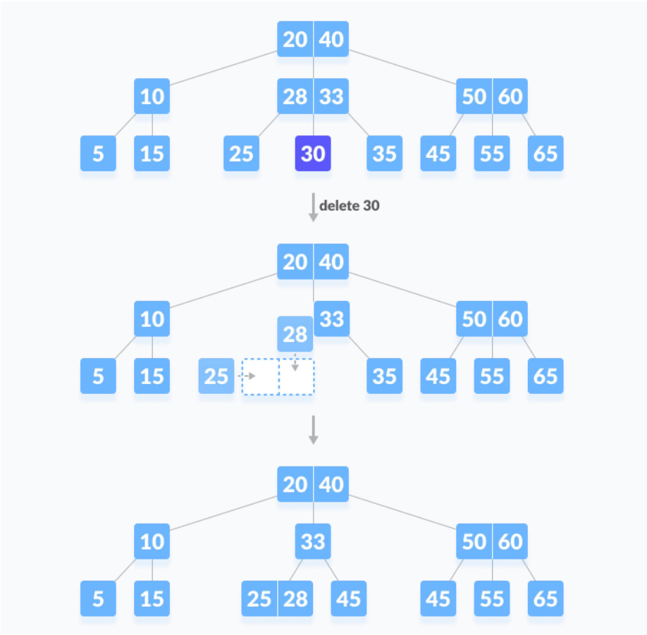
Figure 3.11: Árbol B
