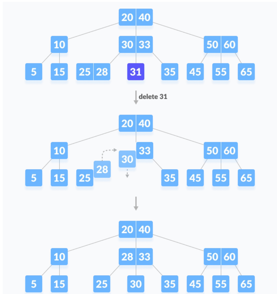
Figure 3.10: Árbol B
