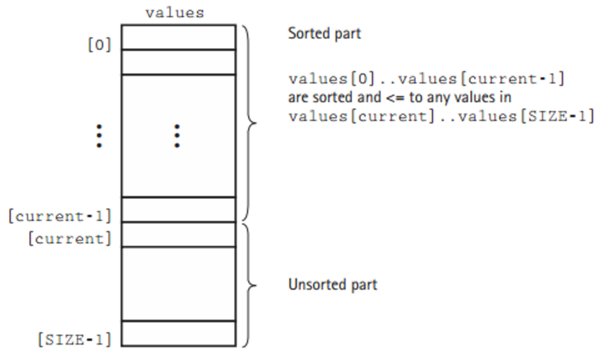
Figure 4.2: División lógica del arreglo
