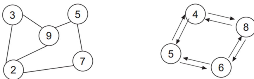
Figure 5.4: grafo conexo y fuertemente conexo
