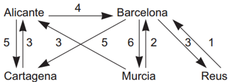
Figure 5.7: matriz grafo ponderado
