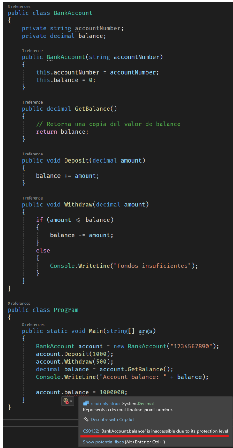
Figure 1.2: Ejemplo de encapsulamiento
