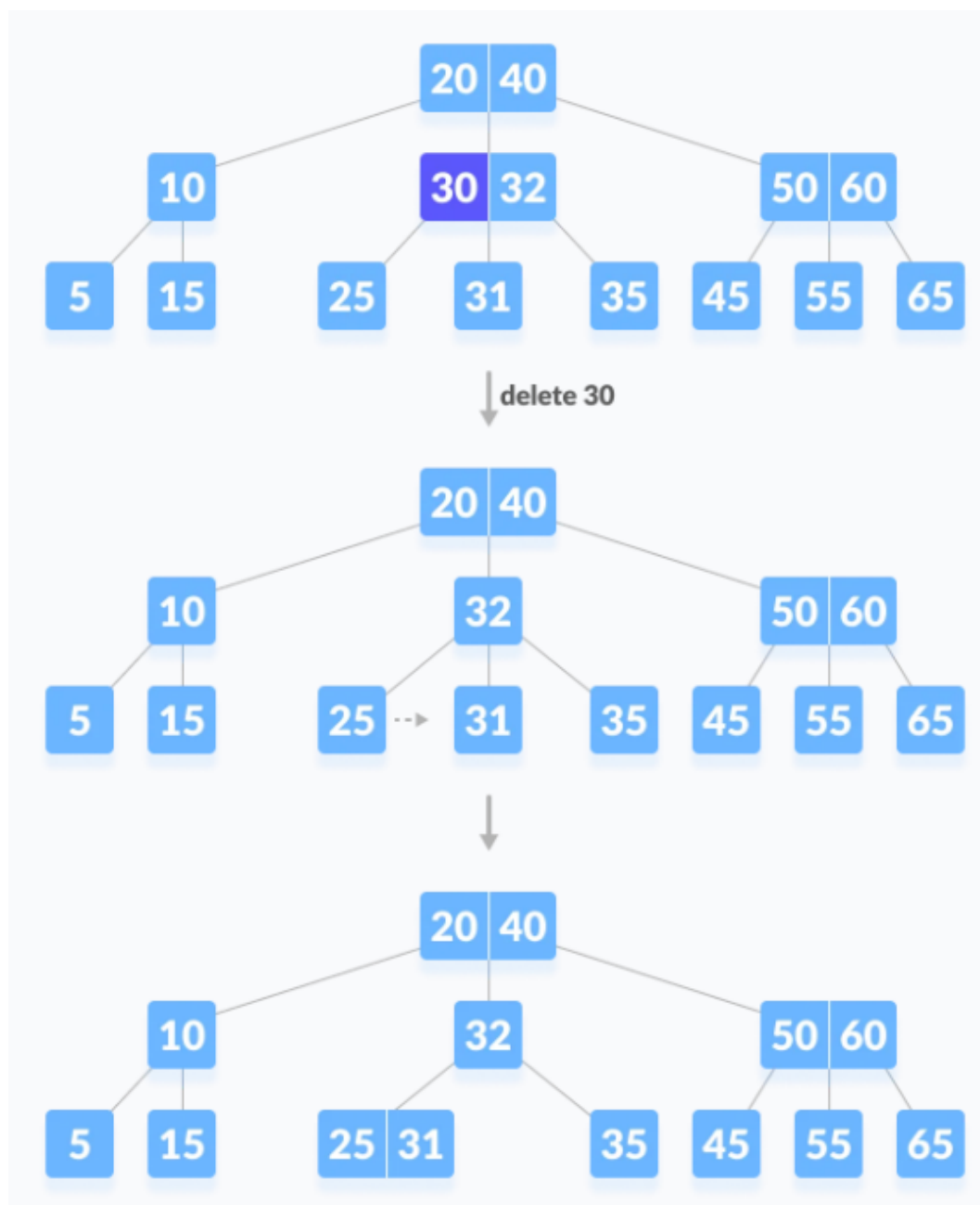
Figura 18: Árbol B
