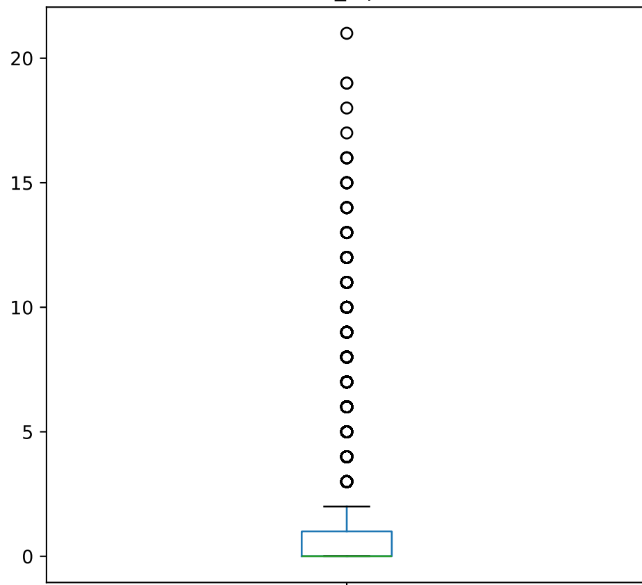
number_inpatient
