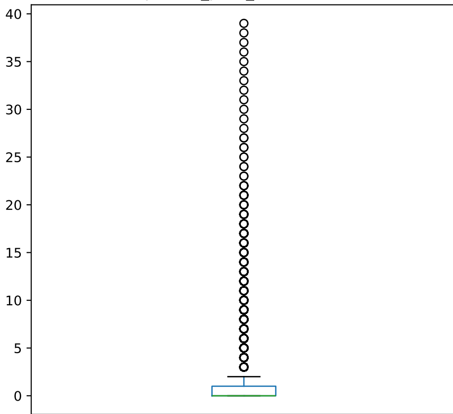
patient_prior_encounters
