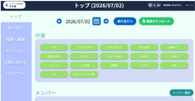
トップ画面
