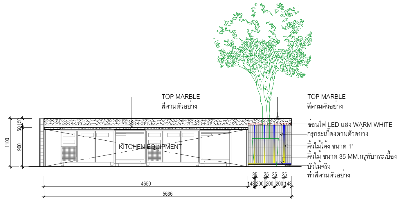
E03 ELEVATION 1 : 50 I-200 COUNTER BAR
