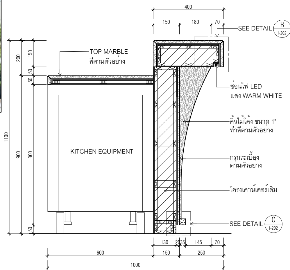
S01 SECTION 1 : 12.5
