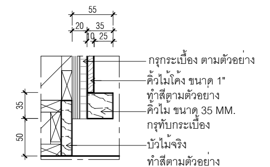
DETAIL C 1 : 5
