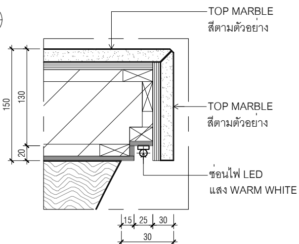
DETAIL B 1 : 5
