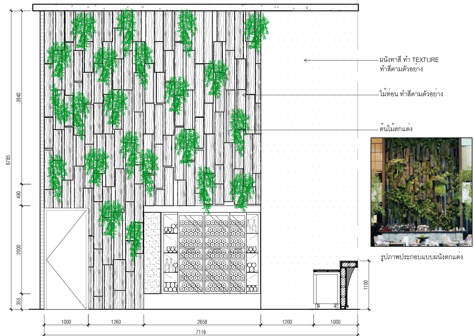
E04 ELEVATION 1 : 50 I-200 COUNTER BAR
