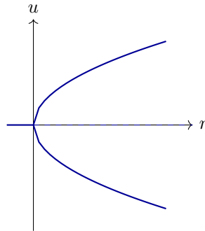
h = 0 Biforcazione Pitchfork
