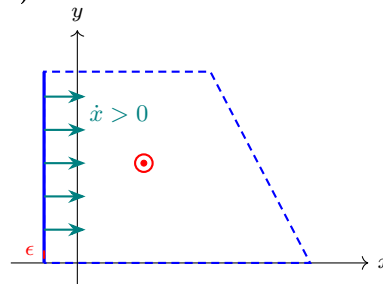
2) Linea x = -\epsilon
