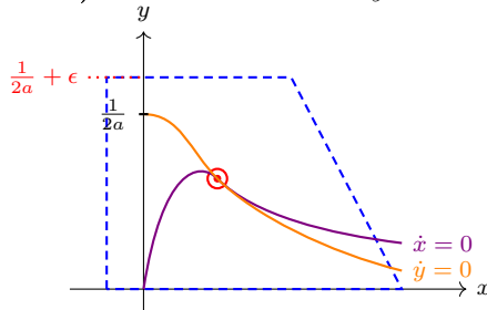
3) Isocline e Max di \dot{y} = 0
