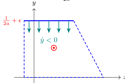
4) Tetto y = \frac{1}{2a} + \epsilon
