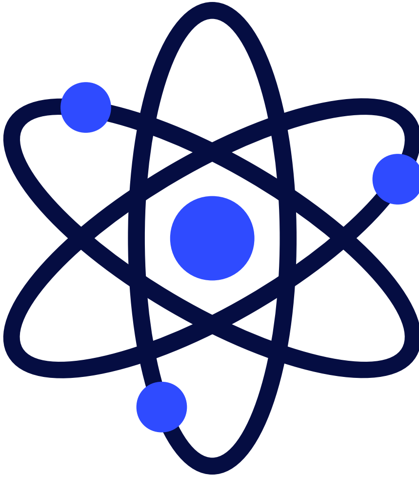
Abbildung 3.2: Beispiel svg
