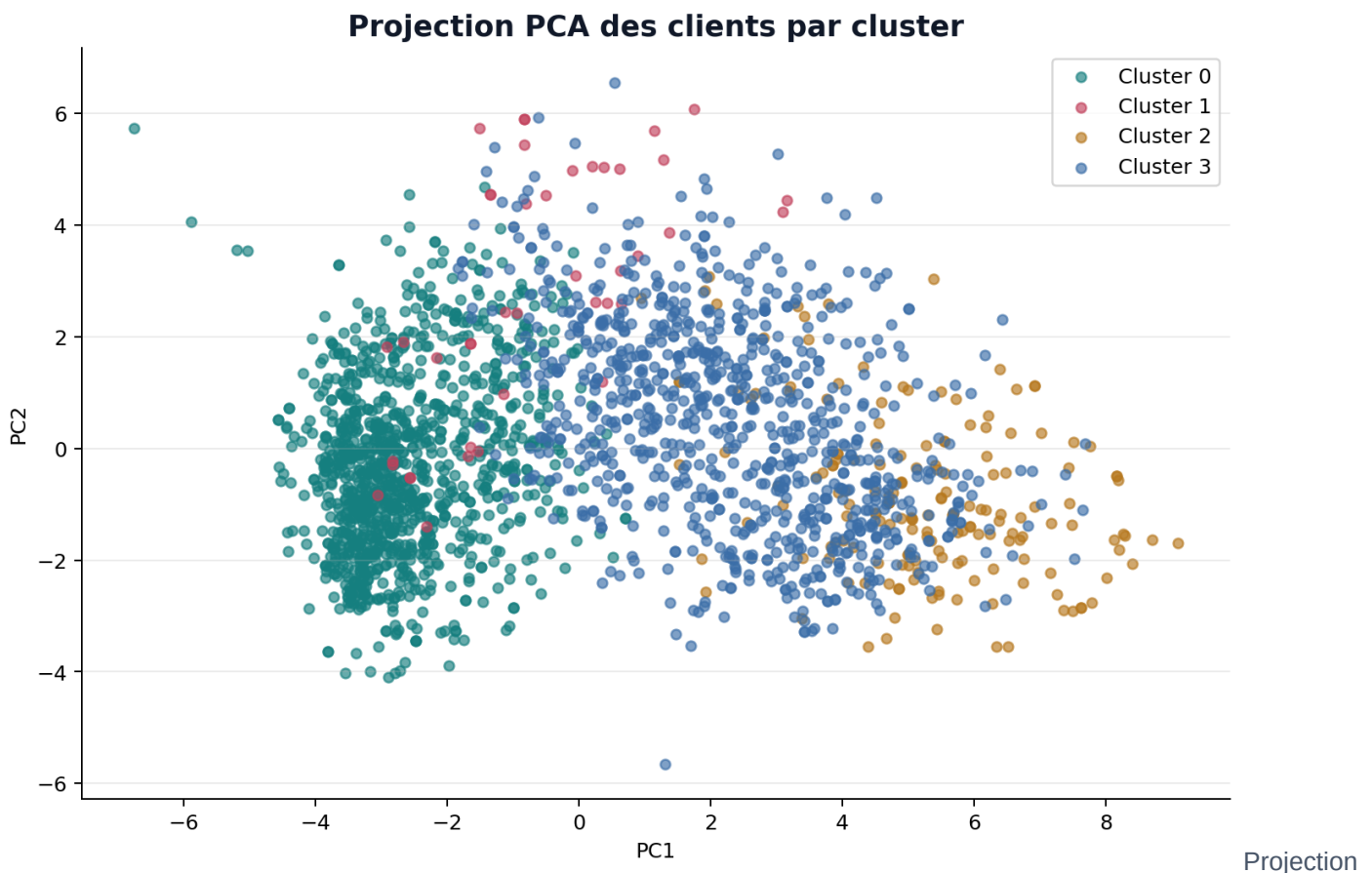
PCA des clients par cluster
