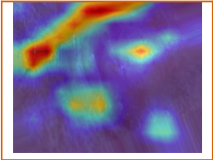
GradCAM++
