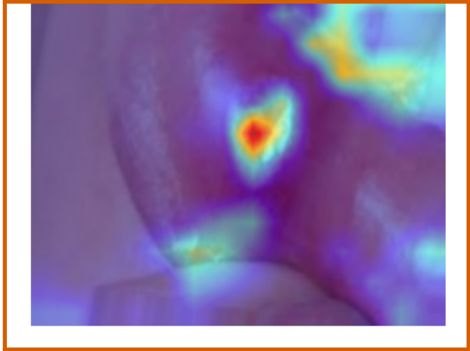
GradCAM++
