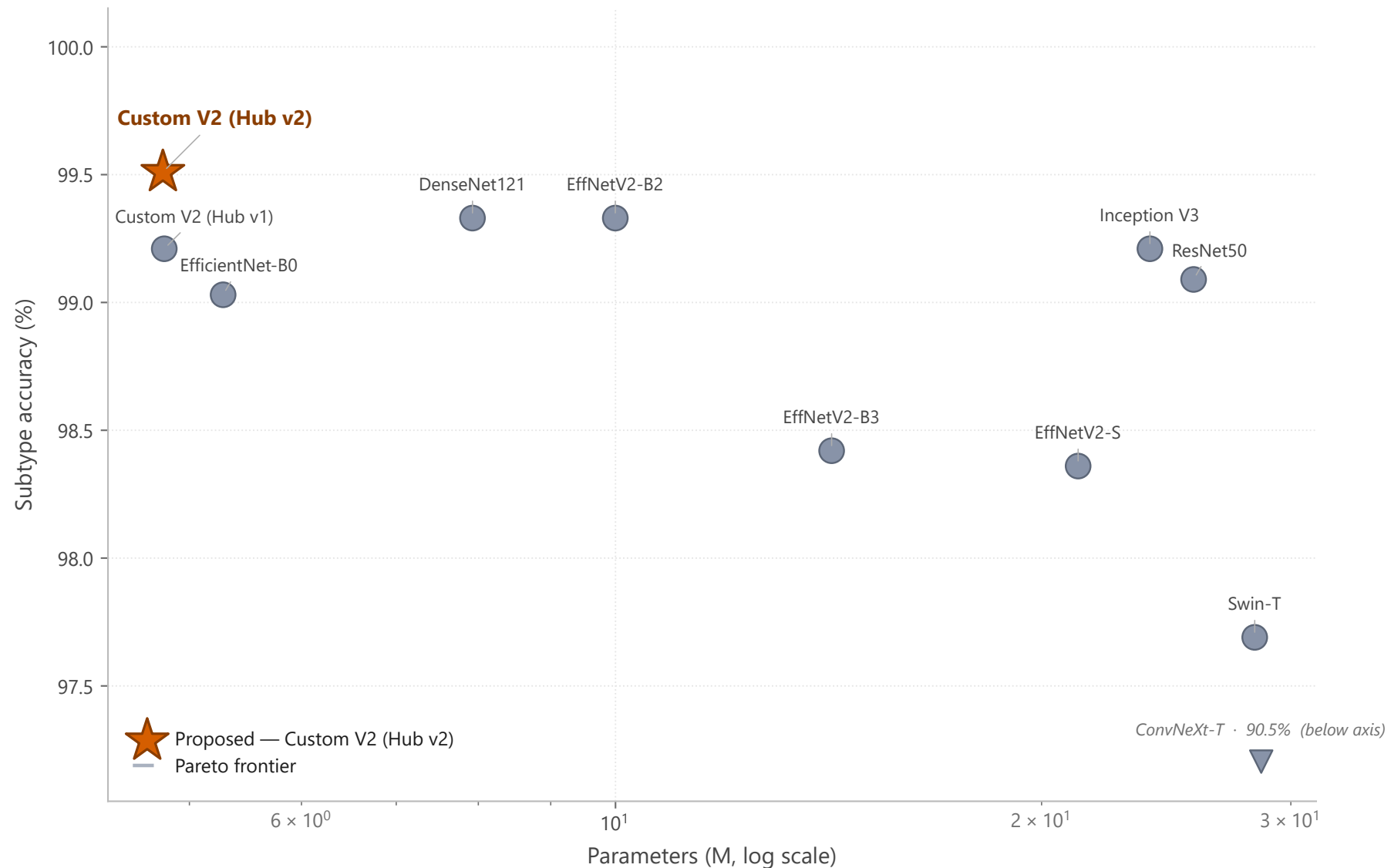
Subtype accuracy vs. parameter count
