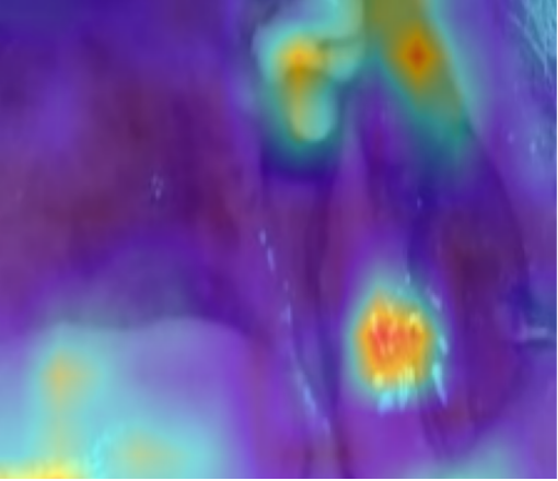
GradCAM++
