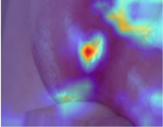
GradCAM++
