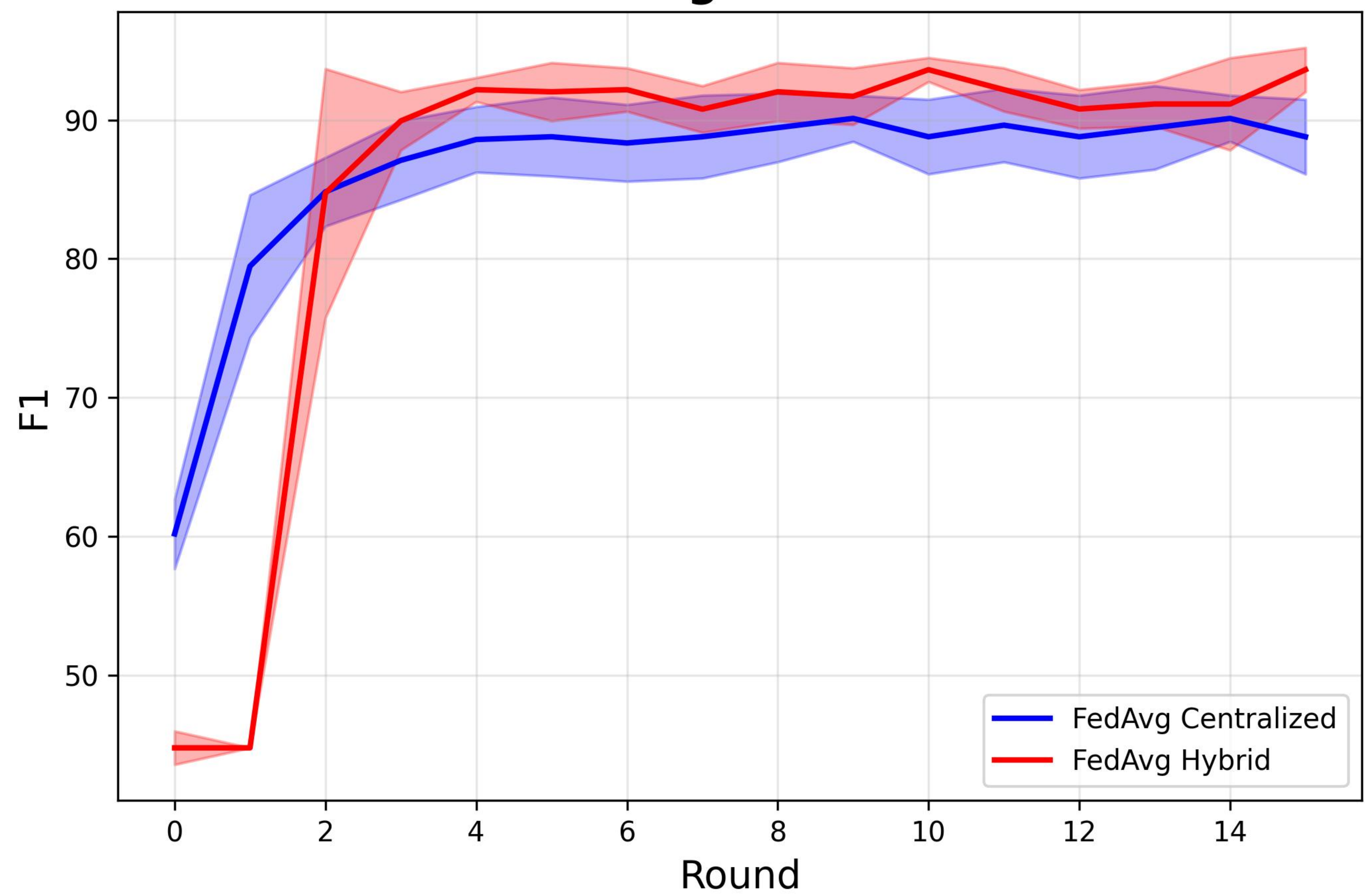
FedAvg F1 score
