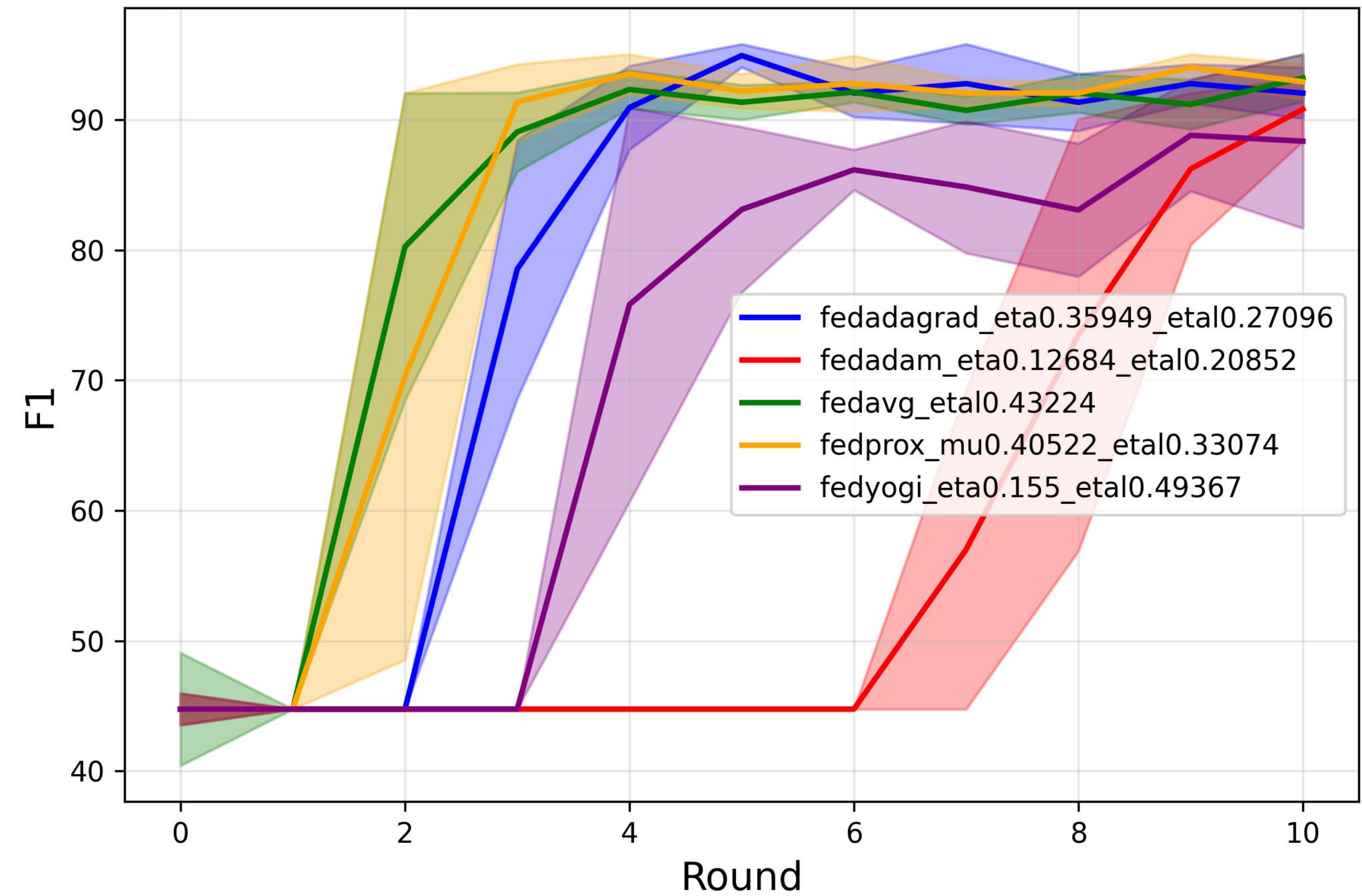
F1 score
