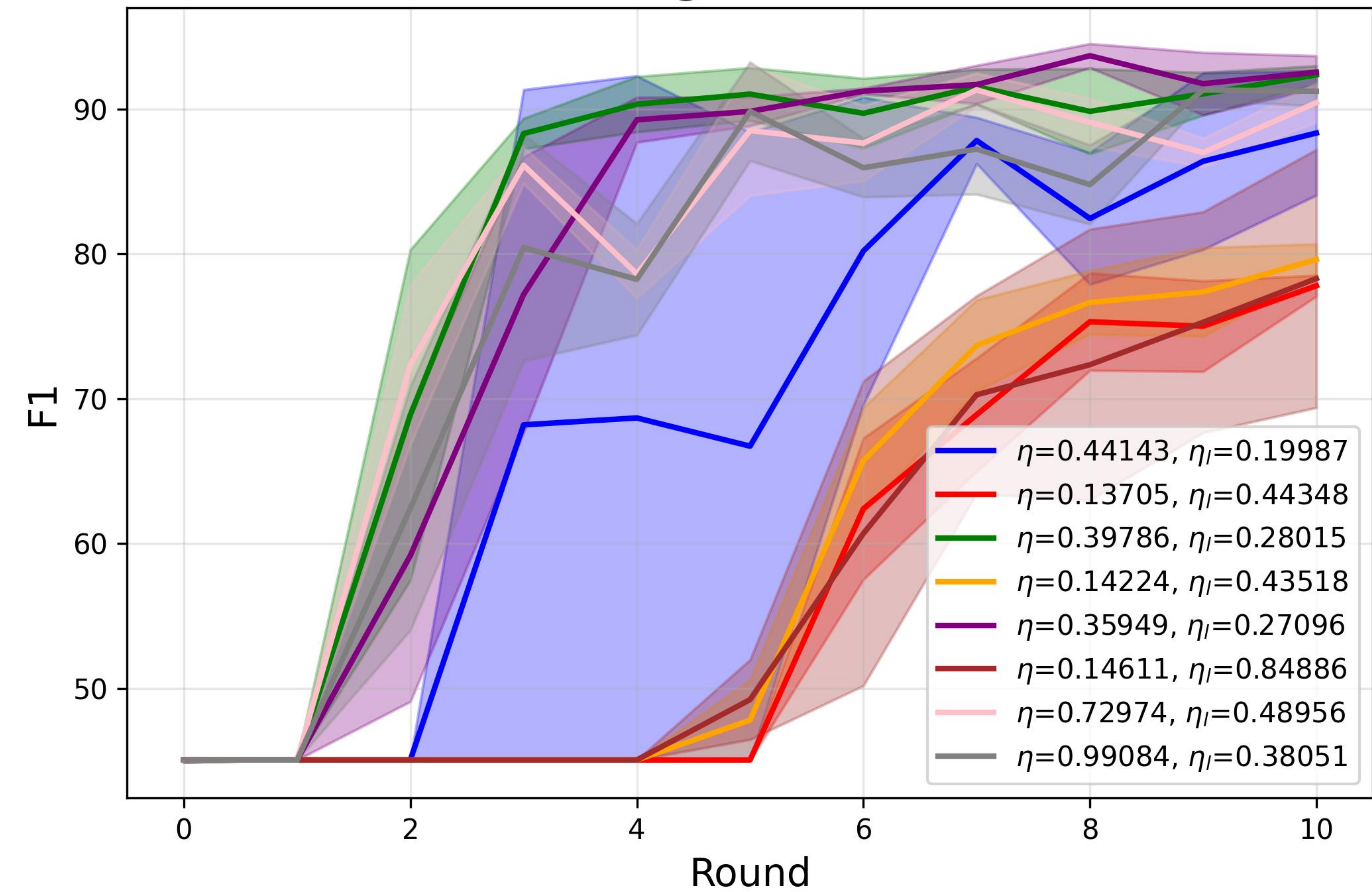
FedAdagrad F1 score
