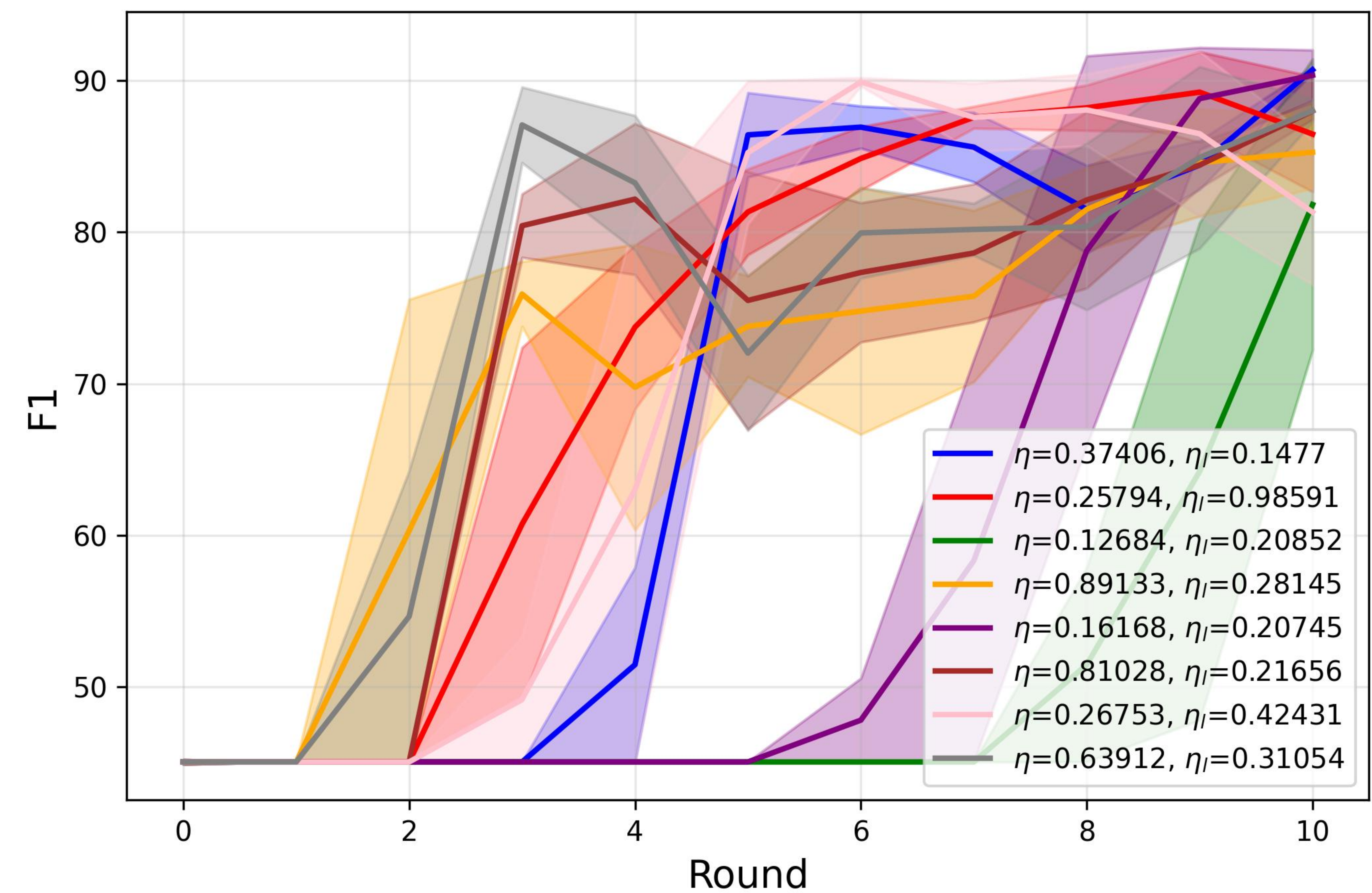
FedAdam F1 score
