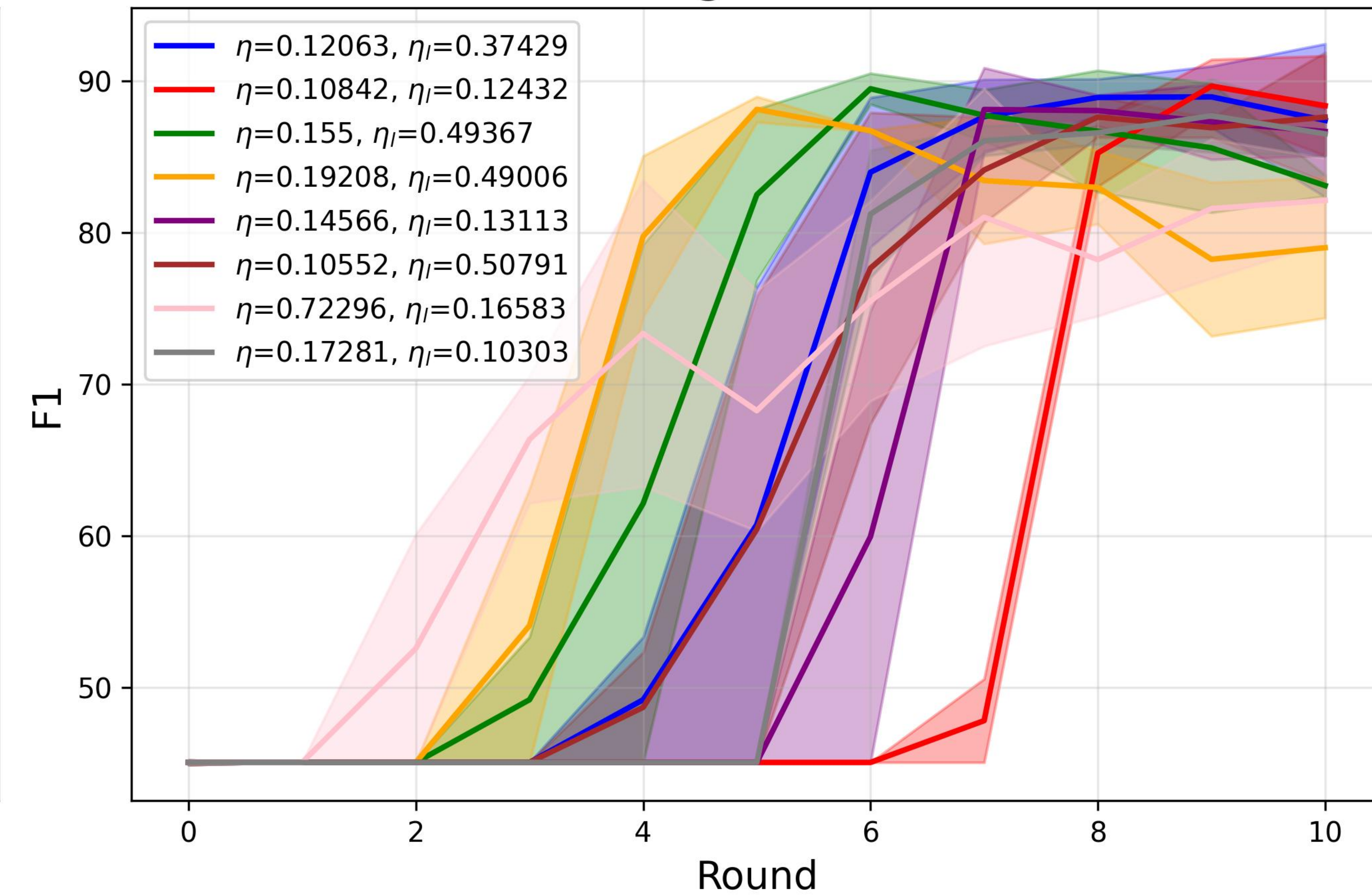
FedYogi F1 score
