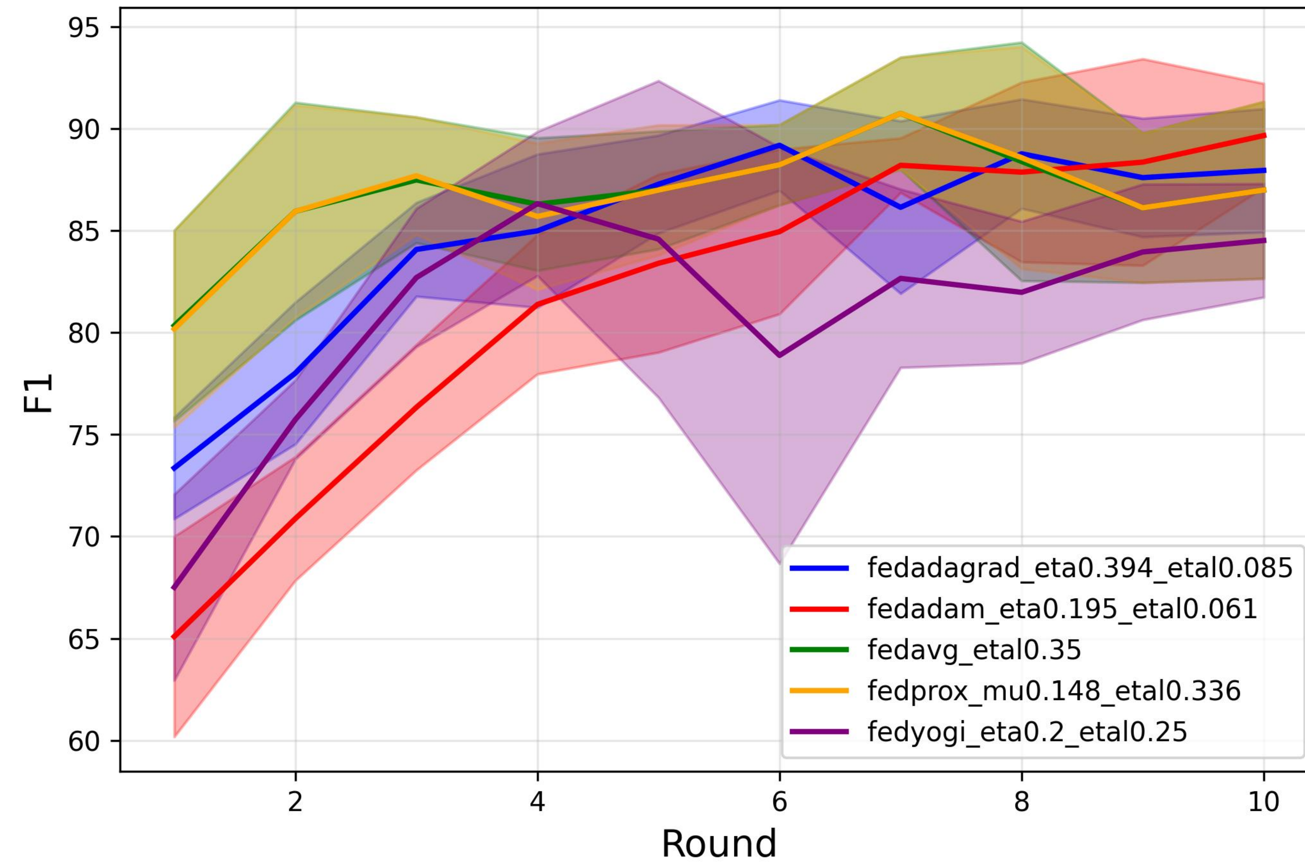
Non-IID Noiseless F1 score
