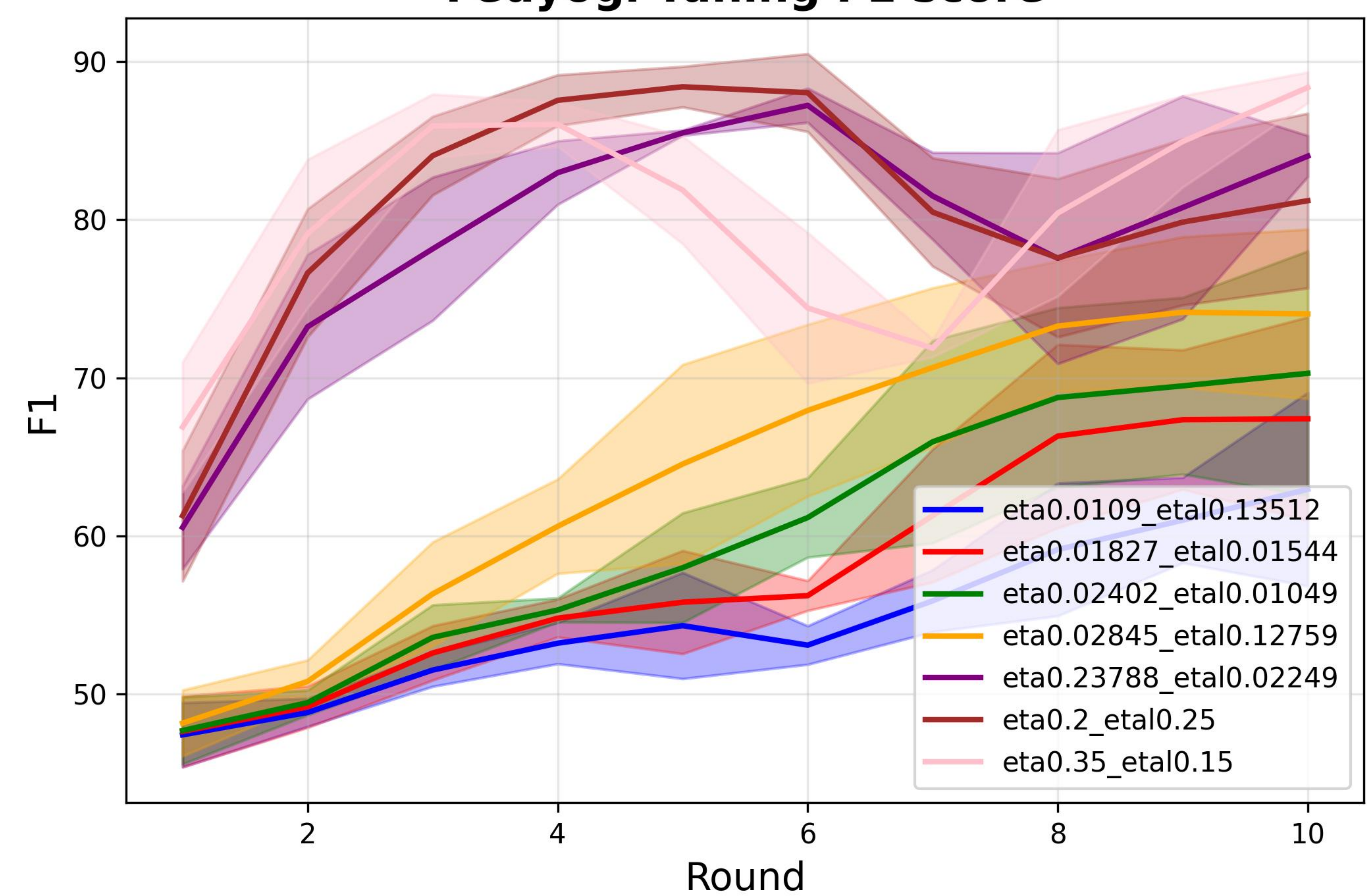
Fedyogi Tuning F1 score
