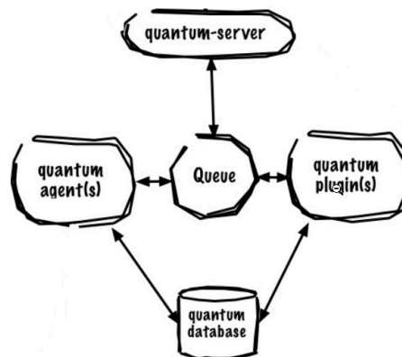
Figure 61 - Neutron (quantum).
