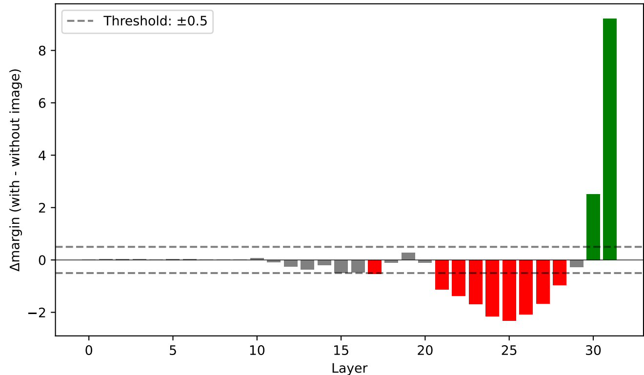
Visual Impact per Layer
