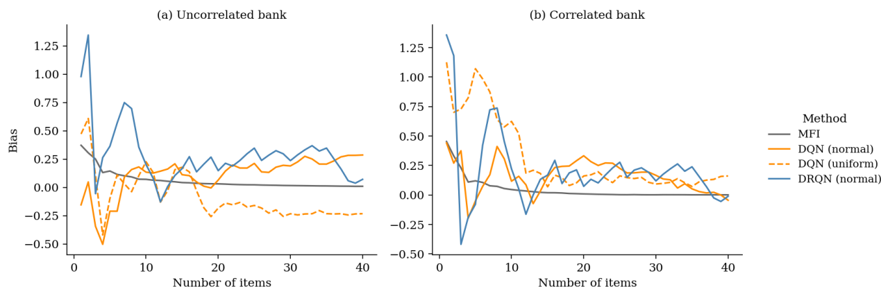
図 7: 各ステップにおける Bias の推移 (無相関バンク・有相関バンク, バンク 1~3 平均)
