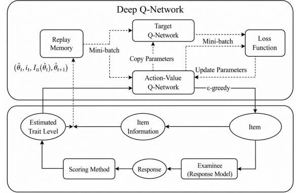
図 4: DQN ベースの項目選択戦略の学習過程. DRQN では状態表現が回答履歴に置き換わり, 経験再生の単位がステップからエピソードへ変更される.
