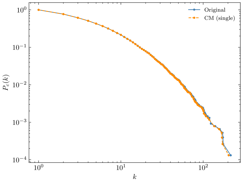
CCDF
