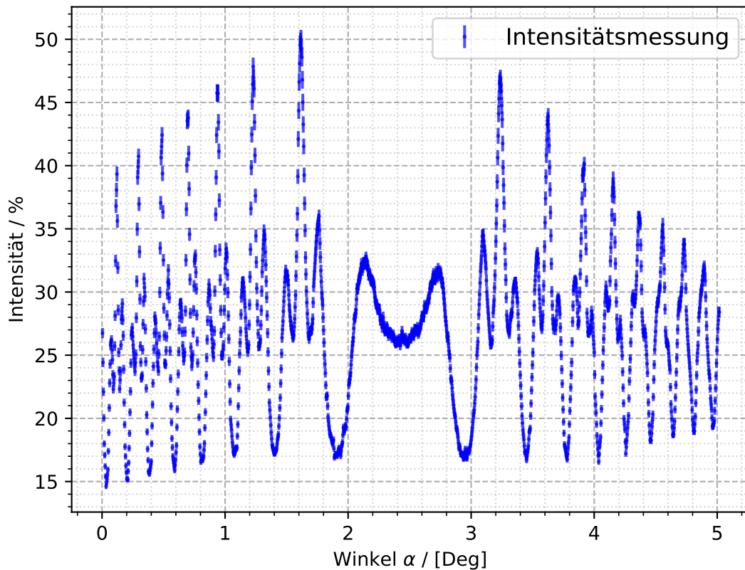
Intensitäten für I = 8,72 \text{ A}
