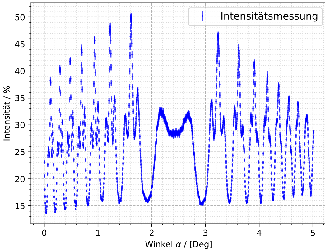
Intensitäten für I = 6,79 \text{ A}
