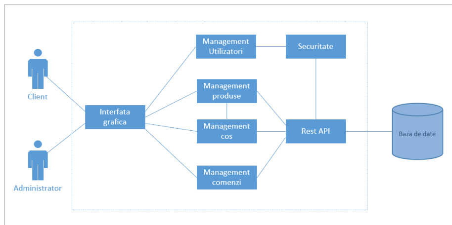
Figure 2: Arhitectura aplicației
