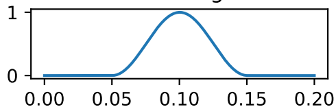
dreptunghi * hanning
