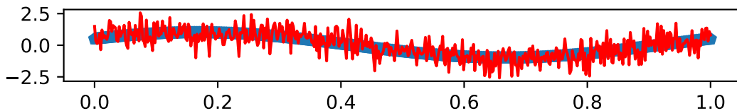
snr: 10
