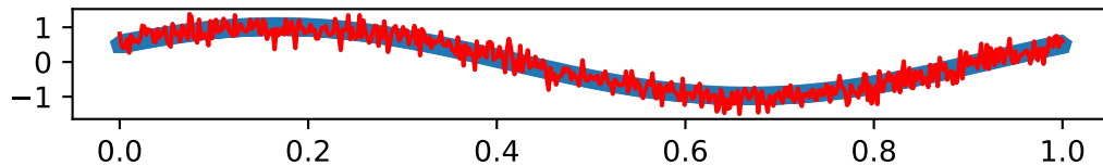
snr: 100
