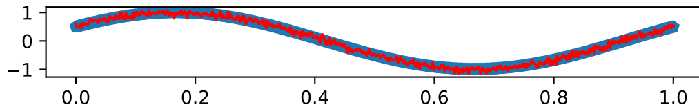
snr: 100
