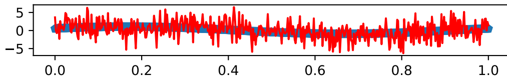
snr: 1
