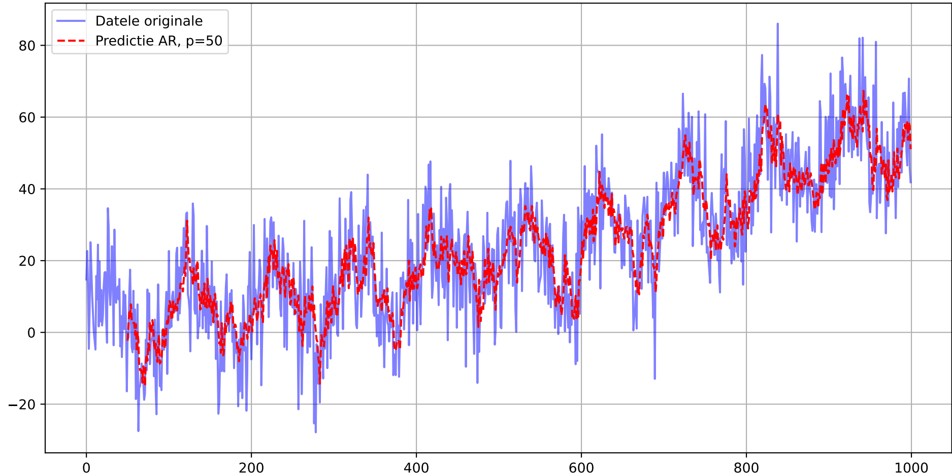
Predictie p=50
