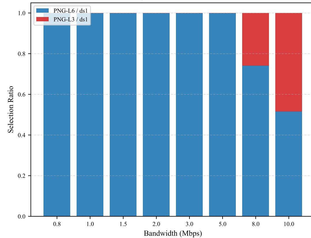
(d) Branch-Migration Pattern Across Bandwidth
