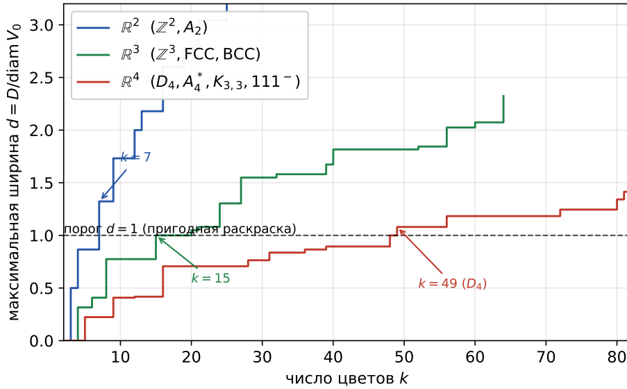
Рис. 2: Максимальная нормированная ширина d(k) как функция числа цветов k для \mathbb{R}^2 , \mathbb{R}^3 , \mathbb{R}^4 (бегущий максимум по классическим решёткам каждой размерности). Пунктир — порог d = 1 : правее точки пересечения раскраска в k цветов правильна для классического расстояния.
