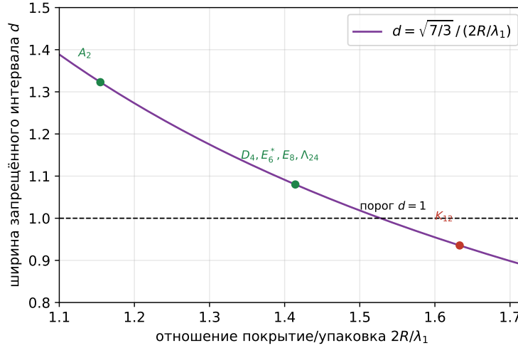
Рис. 5: Тожество (10): ширина d эйзенштейновой конструкции против отношения покрытие/упаковка 2R/\lambda_1 . Проверенные решётки D_4, E_6^*, E_8 (все с отношением \sqrt{2} ) дают ровно d = \sqrt{7/6} ; для \Lambda_{24} положение точки предсказано в предположении (10), а для K_{12} ширина падает ниже порога.
