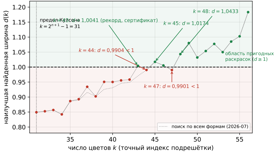
Рис. 4: Наилучшая найденная нормированная ширина d(k) при точном индексе подрешетки k . Зелёные точки ( d \geq 1 ) отвечают пригодным раскраскам, красные — нет. Рекорд — индекс 43 на эйзенштейновой решётке ( d = 1,004111 ); при 44 \leq k \leq 48 показаны оптимумы поиска по всем формам. Немонотонность отражает теоретико-числовую структуру: число доступных подрешёток зависит от разложения k , поэтому «богатые» составные индексы ( 45 = 3^2 \cdot 5 , 48 = 2^4 \cdot 3 ) и эйзенштейновы нормы ( 43 = N(7 + \omega) ) пробиваются легче. Серым — кампания 2026-07 по общим формам, остановившаяся на d \leq 0,990 при k \leq 44 ; пунктир — предел Кулсона k = 31 .
