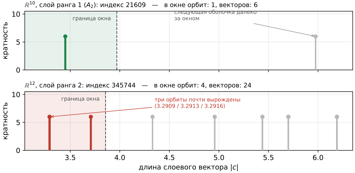
Рис. 8: Длины слоевых векторов подрешётки с кратностями. Сверху слой ранга 1 (размерность 10): в окне одна орбита, следующая оболочка далеко. Снизу слой ранга 2 (размерность 12): четыре орбиты, три почти вырождены.
