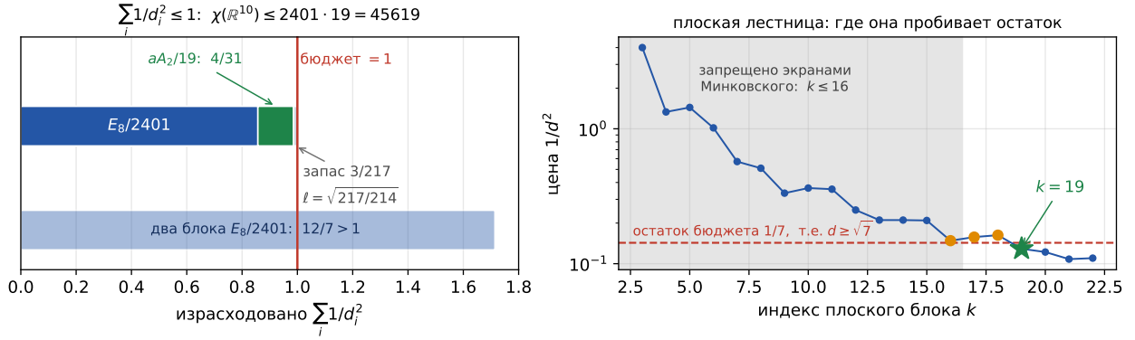
Рис. 6: Слева: бюджет \sum_i 1/d_i^2 \leq 1 как полоса длины 1. Блок E_8/2401 занимает 6/7 , плоский проставок индекса 19 — 4/31 , остаток 3/217 и даёт ширину \ell = \sqrt{217/214} . Два блока E_8/2401 в бюджет не помещаются ( 12/7 > 1 ) — поэтому в произведении может быть лишь один эффективный блок. Справа: плоская лестница цены 1/d^2 по индексу; горизонталь — остаток бюджета 1/7 , серая зона запрещена экранами (§9.4).
