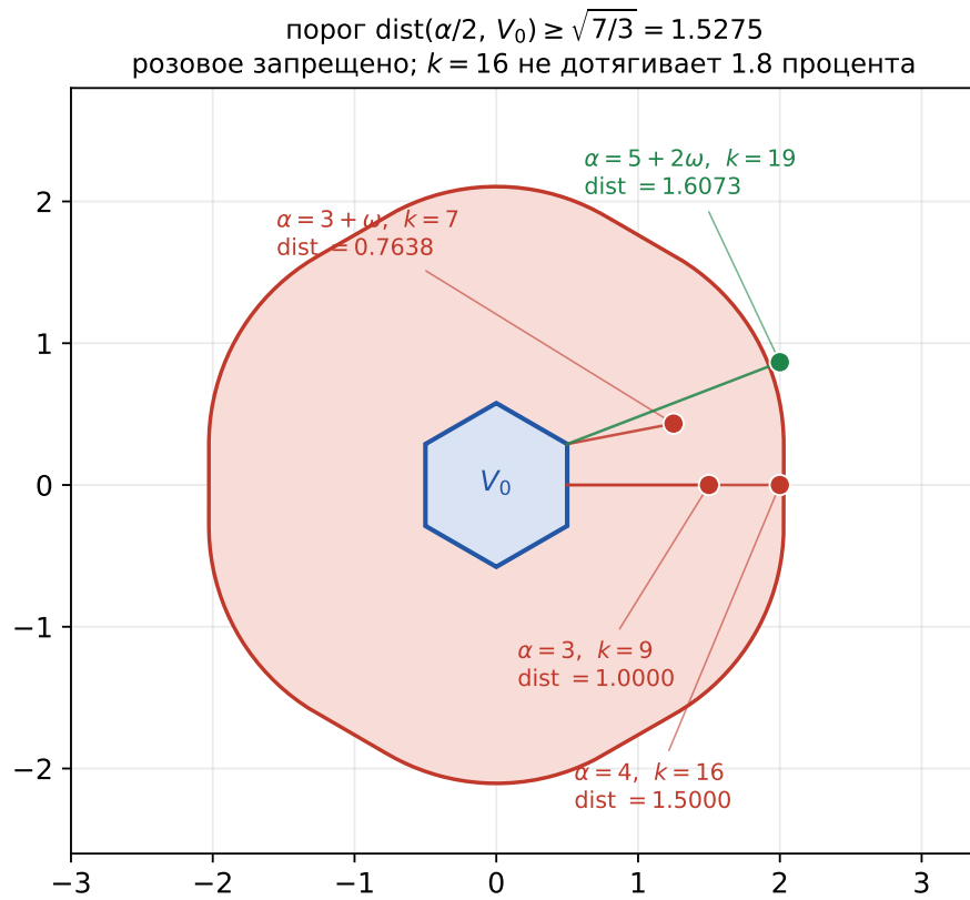
Рис. 7: Почему плоский проставок стоит ровно 19. Синий шестиугольник — ячейка V_0 решётки A_2 ; розовая область — её окрестность радиуса \sqrt{7/3} = 1,5275 , куда точка \alpha/2 попадать не должна. Отрезки ведут к ближайшей точке ячейки. Индекс 16 ( \alpha = 4 ) не дотягивает 1,8%, и лишь \alpha = 5 + 2\omega выходит наружу.
