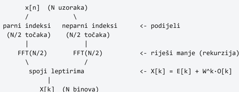
Slika 2. «Podijeli pa vladaj»: \log_2 N razina, svaka N/2 leptira \rightarrow N \cdot \log_2 N operacija.
