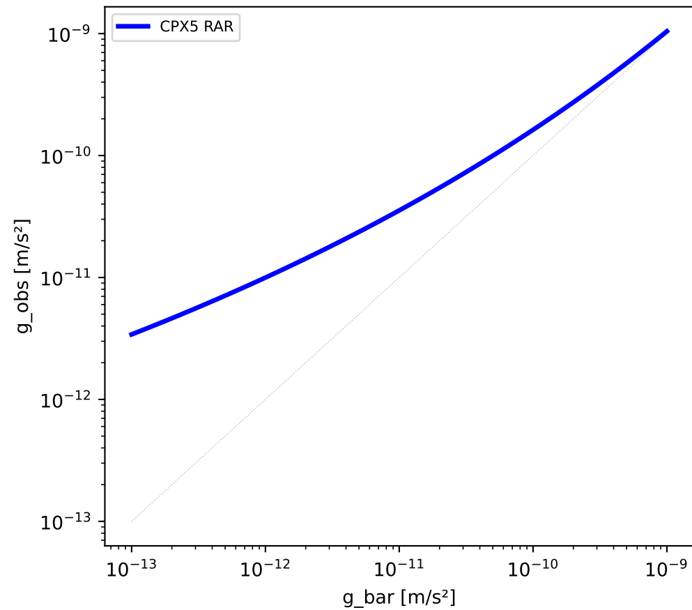
(b) Universal CPX5 RAR
