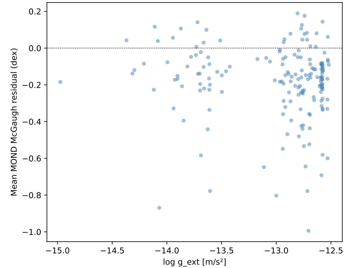
Per-galaxy: \rho=-0.1060 ( p=1.62\text{e-}01 )
