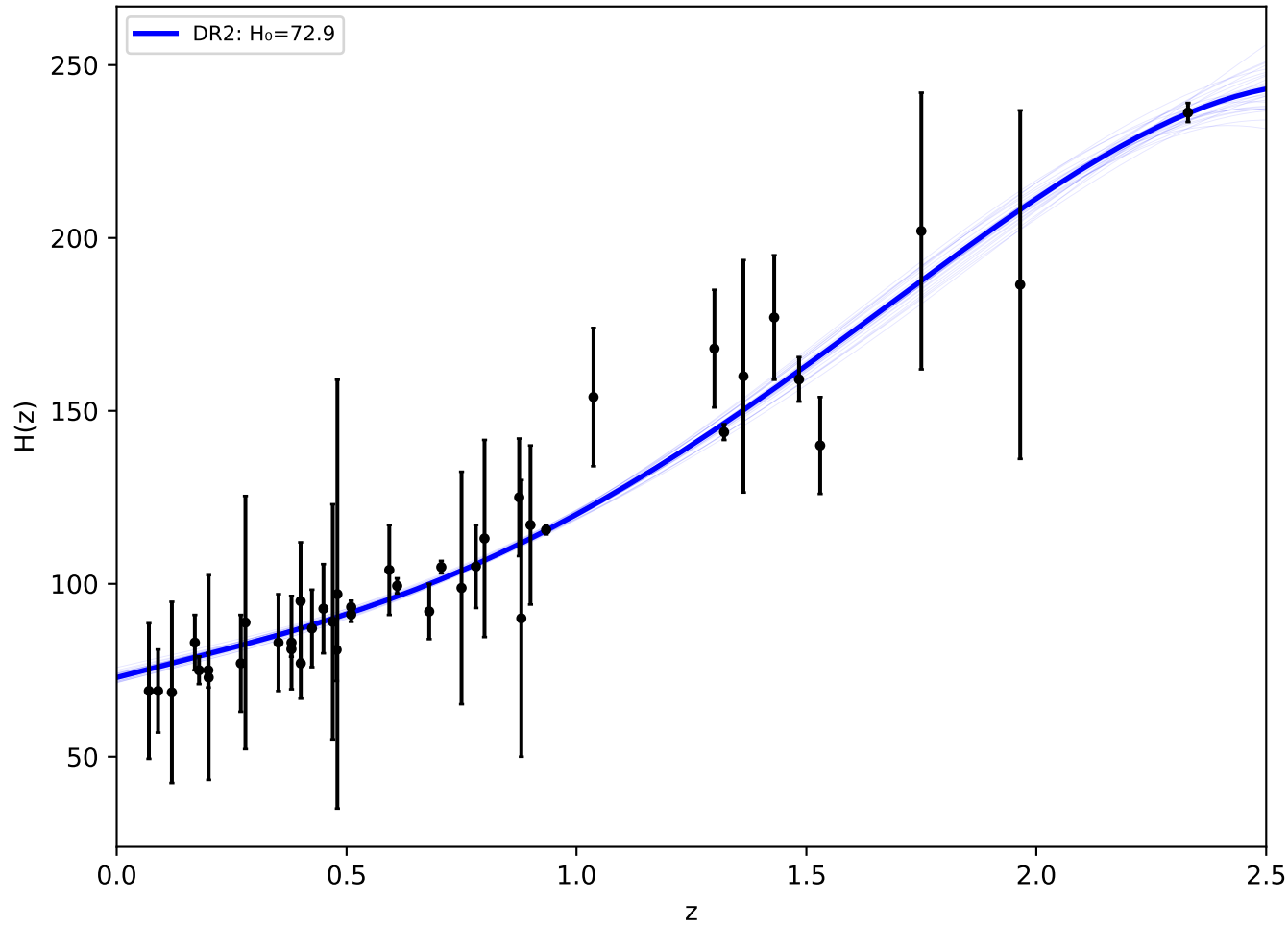
H(z) data + Cpx 13 fit
