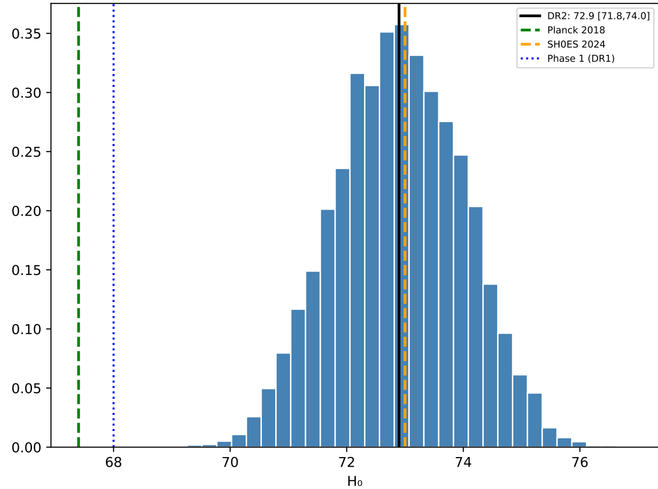
H_0 Posterior
