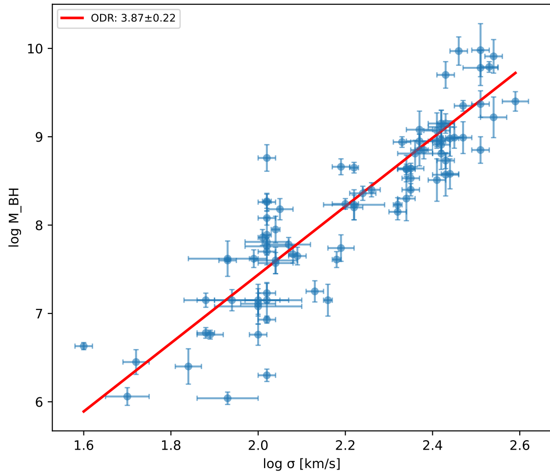
M-sigma
