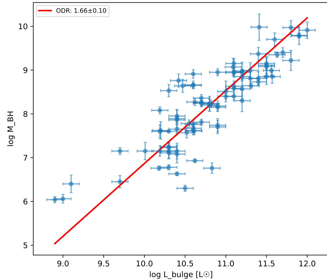
M-L
