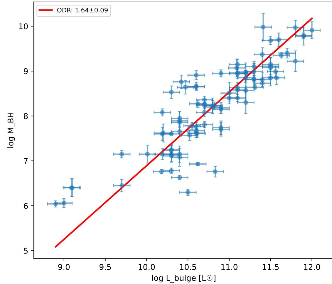
M-L: \chi^2_{\text{red}}=12.7
