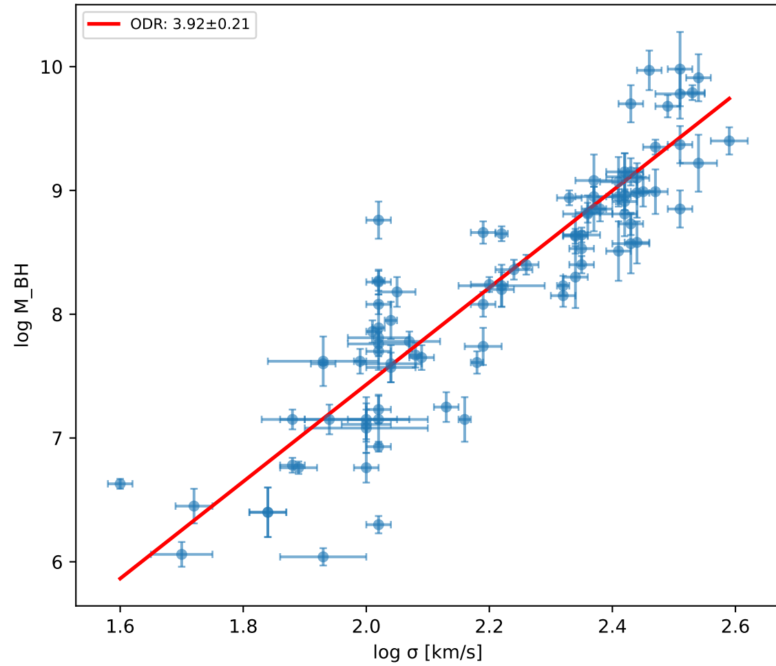
M-sigma: \chi^2_{\text{red}}=23.8
