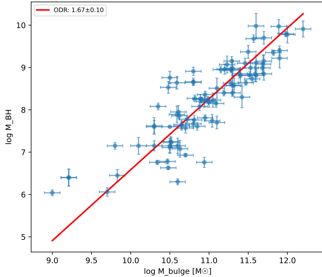
M-M_bulge: \chi^2_{\text{red}}=12.3
