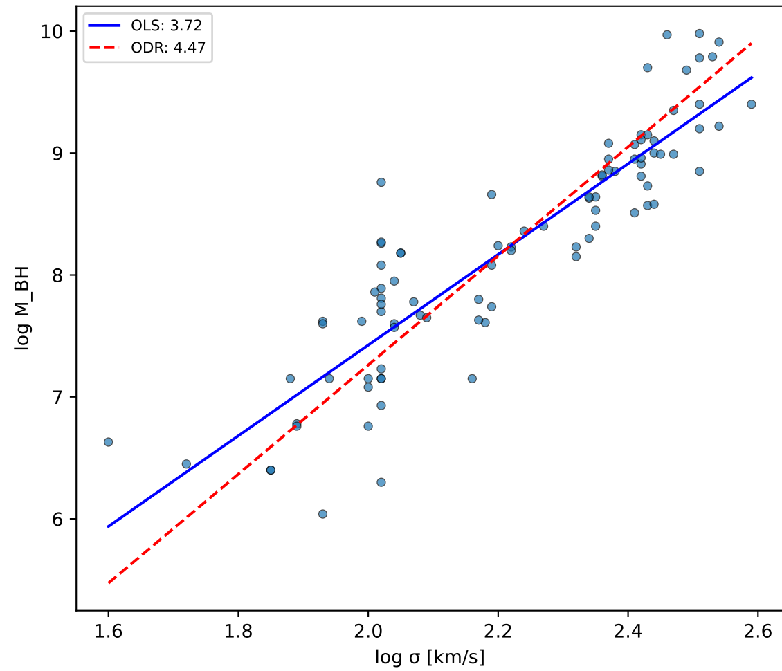
M-sigma: RMS=0.417
