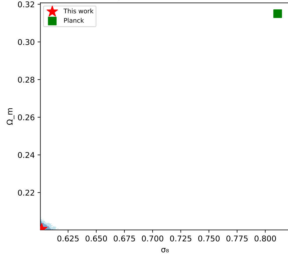
(c) Joint VF+SMF Posterior
