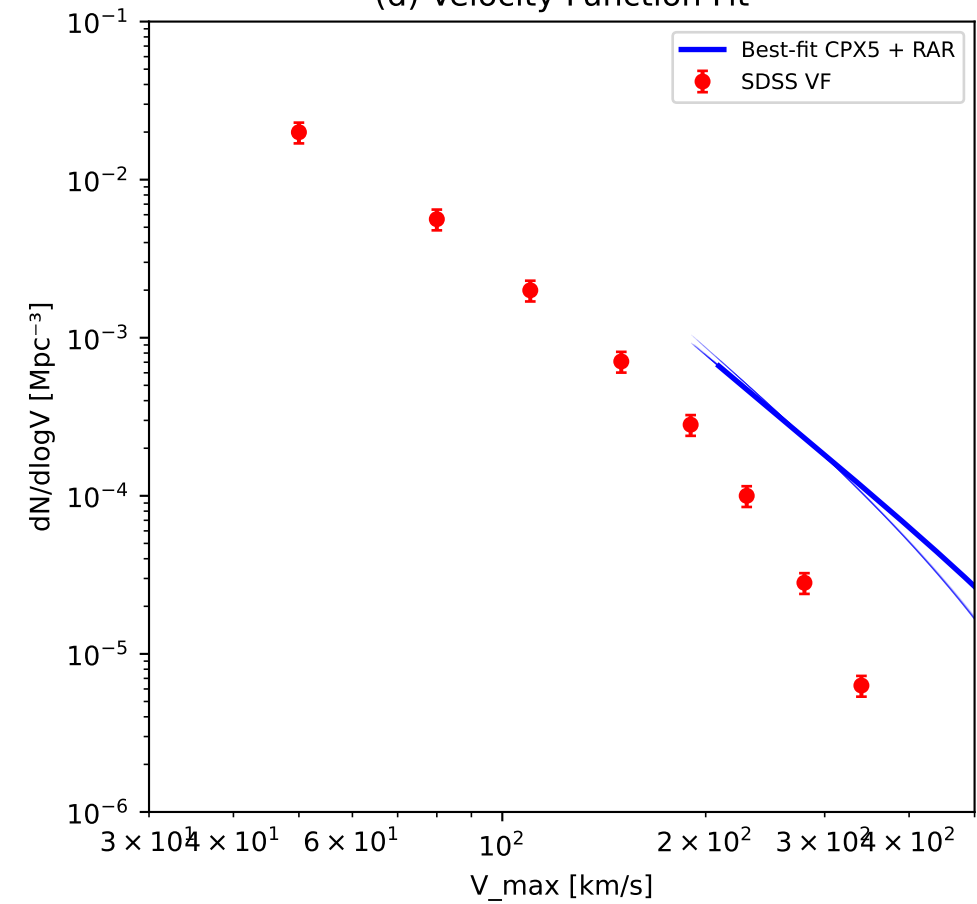
(d) Velocity Function Fit
