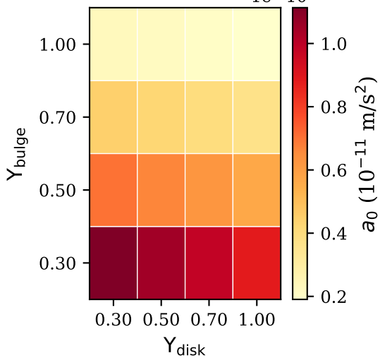
(d) MOND a_0 vs M/L ( 5.8 \times range)
