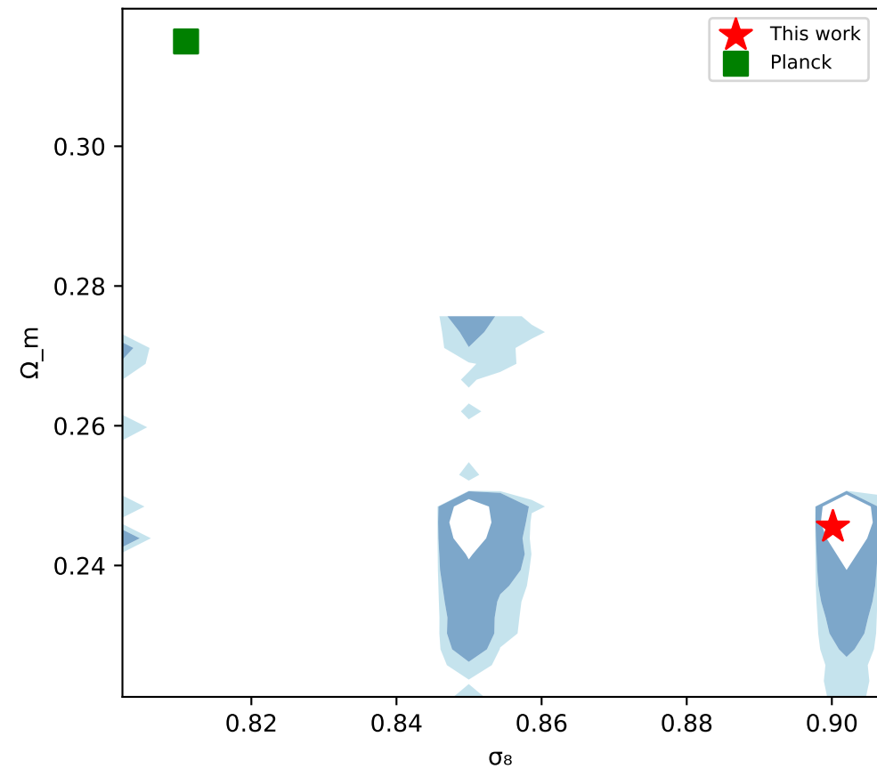
(c) Posterior ( \sigma_8=0.90 \pm 0.03 )
