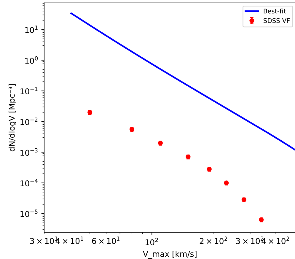
(a) VF — Abundance Matching
