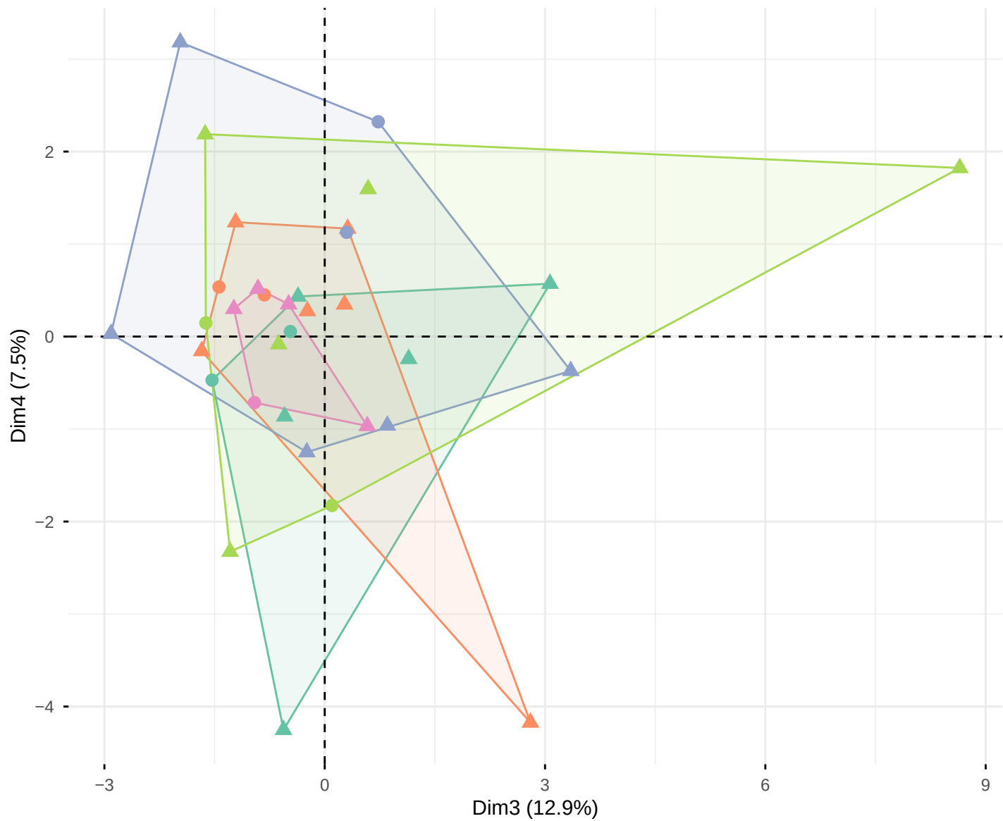
PC 3&4 – all parameters
