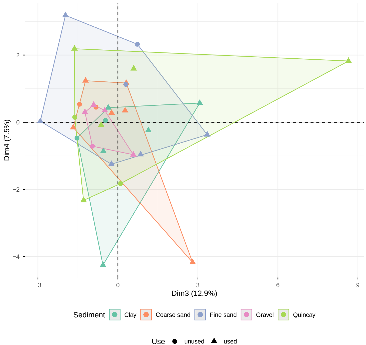
PC 3&4 – all parameters
