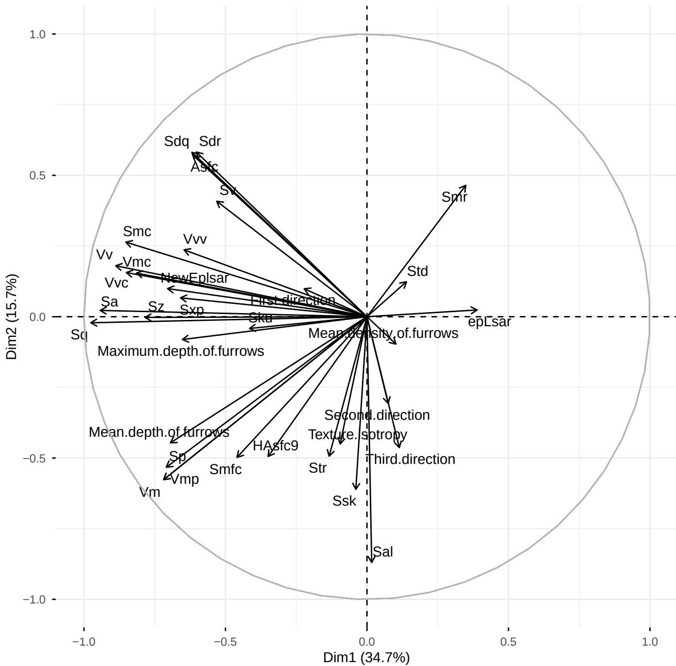
PC 1&2 – all parameters
