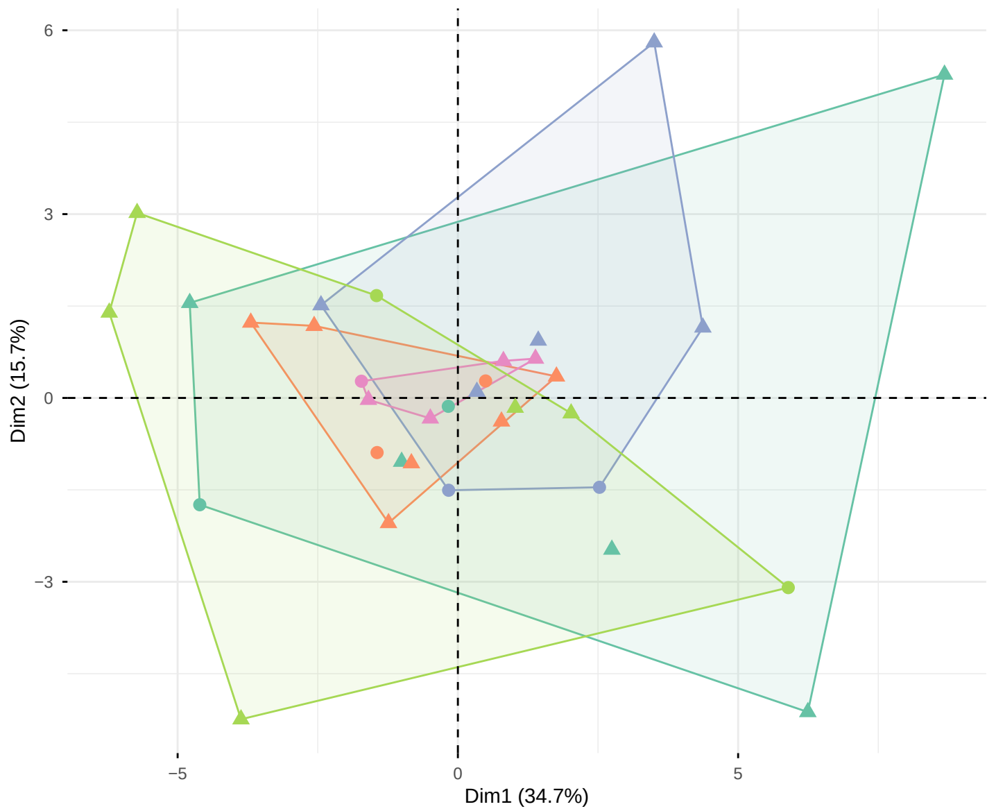
PC 1&2 – all parameters
