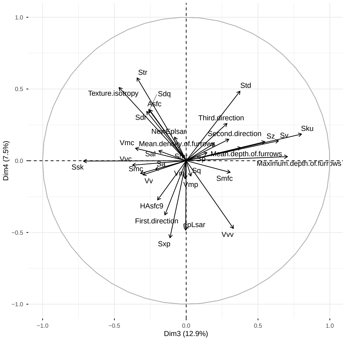
PC 3&4 – all parameters
