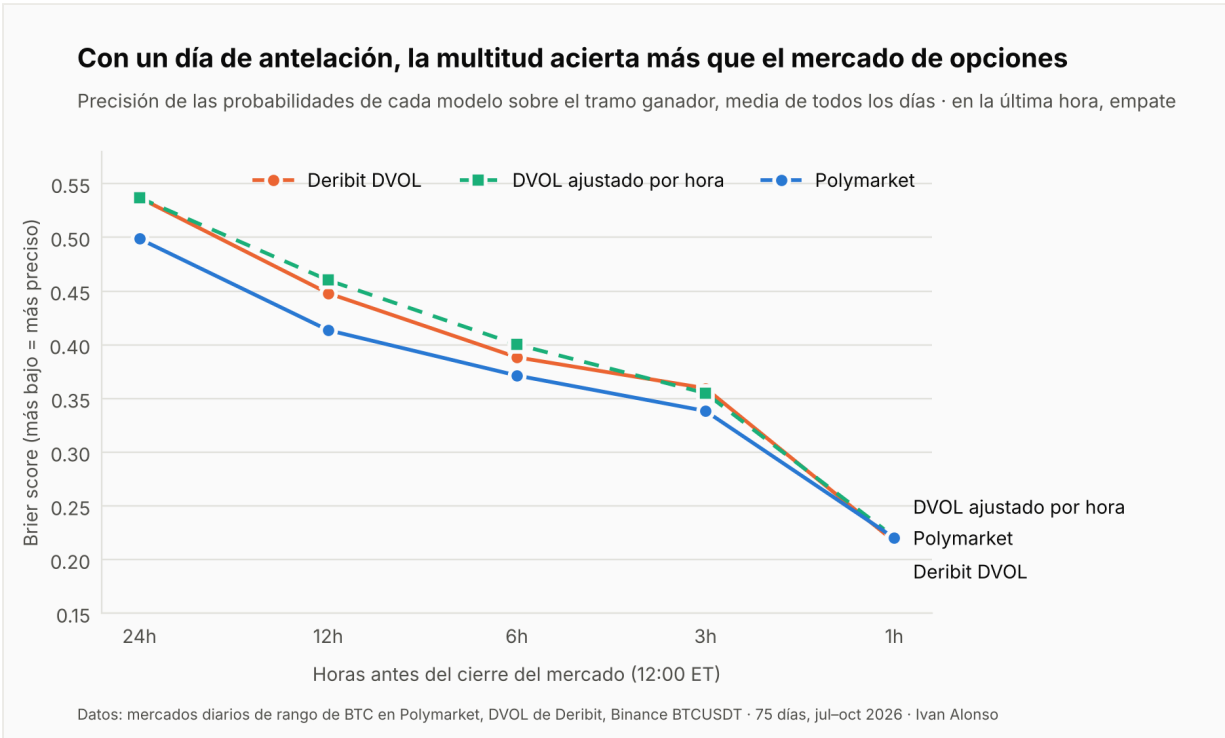
Figura 2. Precisión de cada modelo según las horas al cierre.
