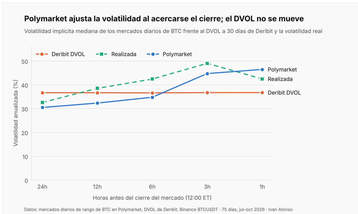
Figura 1. Volatilidad implícita mediana de Polymarket frente al DVOL y a la volatilidad que realmente hubo, según las horas al cierre.
